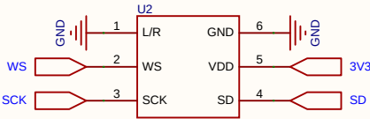
Micrófono INMP441
